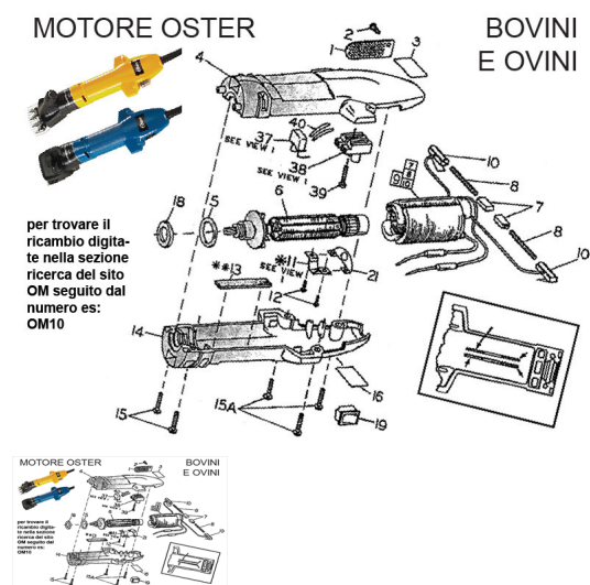
RICAMBIO OSTER OV/BO STATORE FIG. OM9
