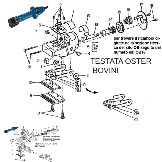
RICAMBIO OSTER BOVINI VITE FISSA BLOCC PRESS FIG. OB2
