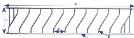
Barriera con tubo obliquo per vitelli
