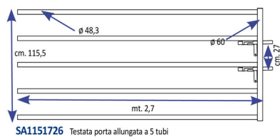
SA1151726 Testata porta allungata a 5 tubi
