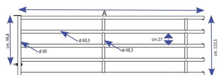
Barriera a 5 tubi con testata femmina
