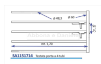
SA1151714 Testata porta a 4 tubi
